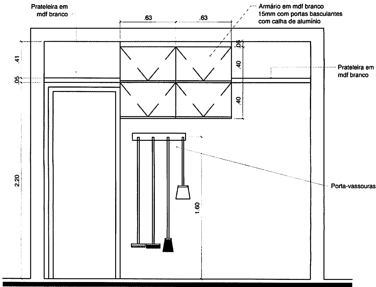
VISTA FRONTAL ARMÁRIO - LANCHONETE ESCALA:.....1/25
