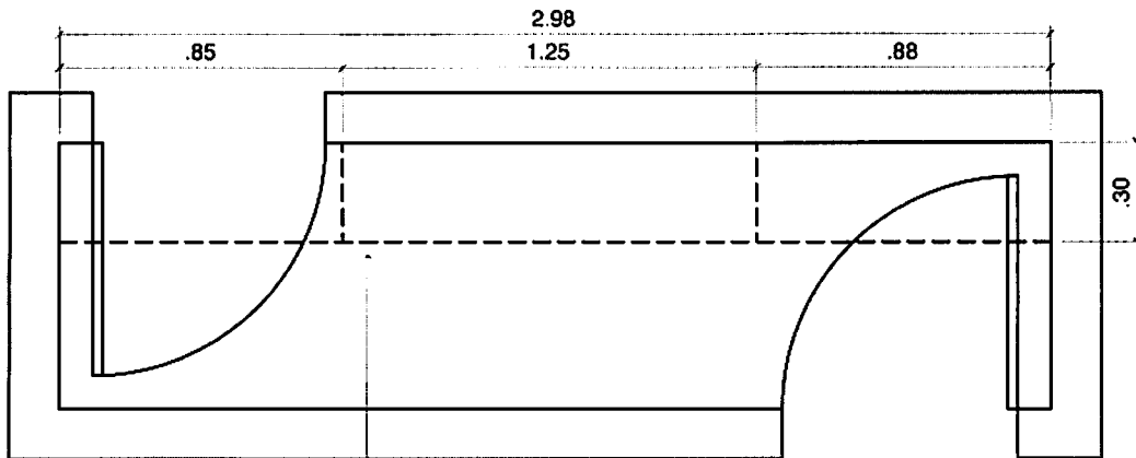
PLANTA BAIXA ARMÁRIO - LANCHONETE ESCALA:.....1/25
